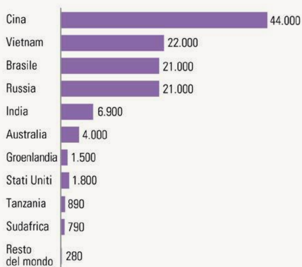
Figura 51 Disponibilità mondiale dei minerali del gruppo terre rare (tonnellate)
