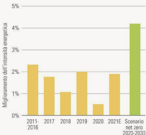
Figura 49 Miglioramenti globali dell'intensità energetica nel decennio 2011-2021
