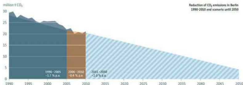
Riduzione delle emissioni di CO 2 a Berlino tra il 1990-2010 e scenario di riduzione al 2050
